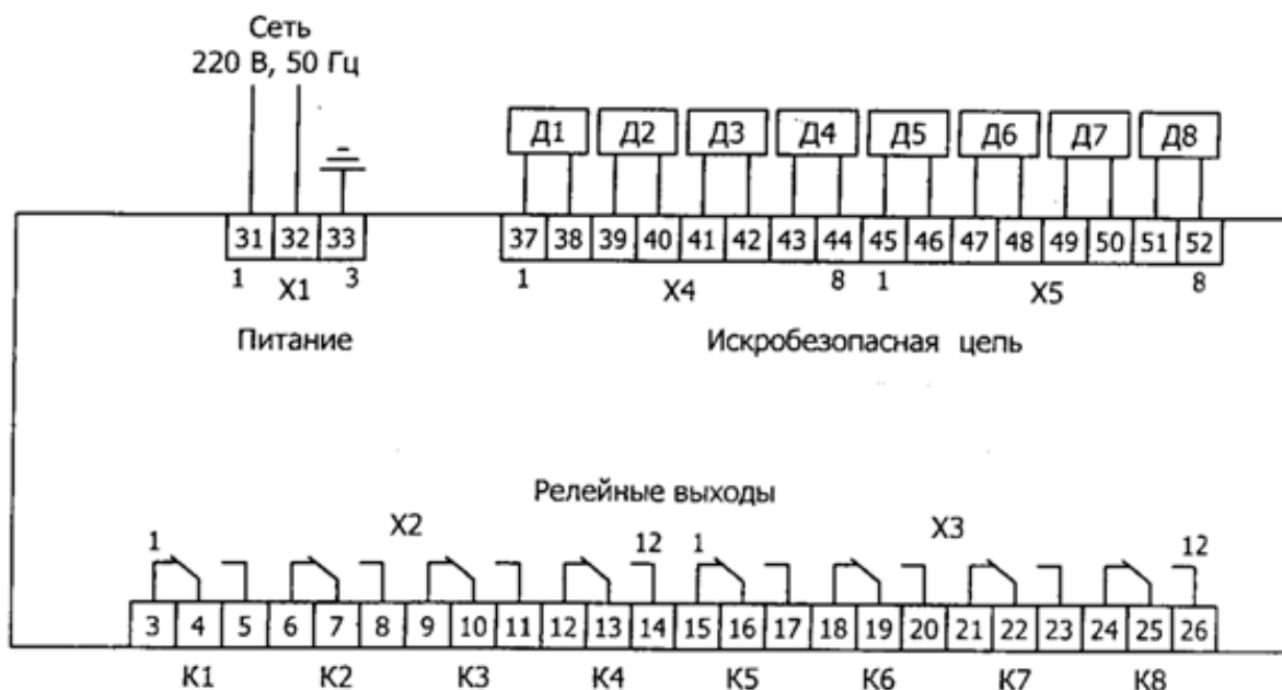
Рис.1 Схема подключения.
