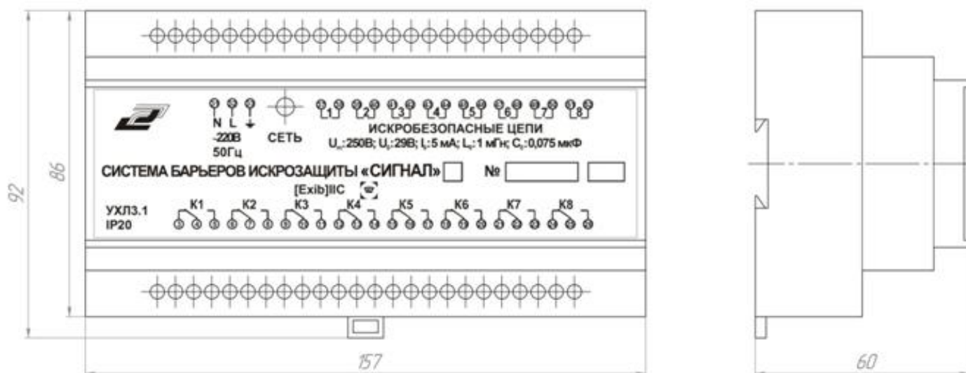
Рис.2 Габаритные размеры системы барьеров искрозащиты «Сигнал»
