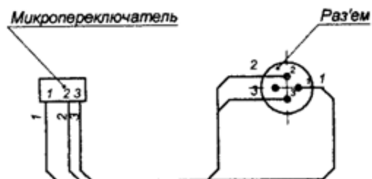
Рис. 2. Схема электрического подключения
